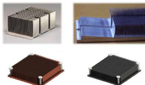
Folded Fin / Skived Fin
